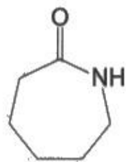
caprolactam
